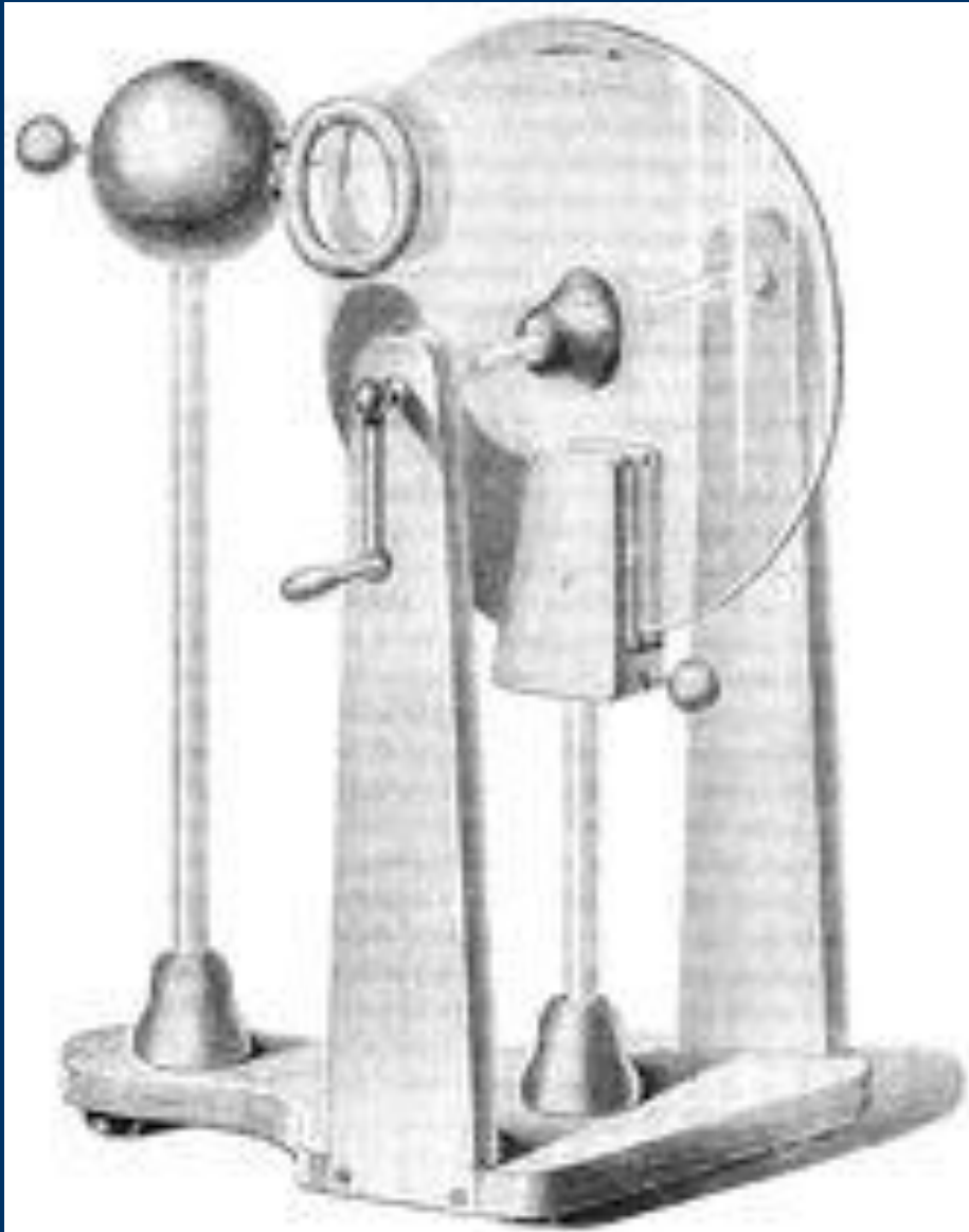
Winter-féle dörzselektromos gép (1850)
